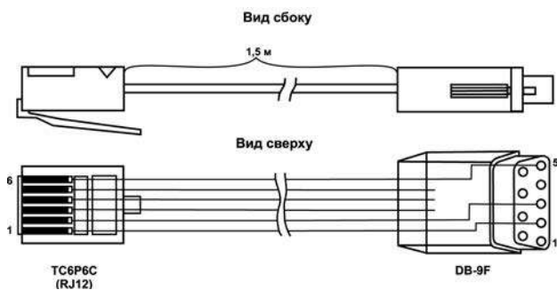
Рисунок Д.2 – Схема кабеля КС2
