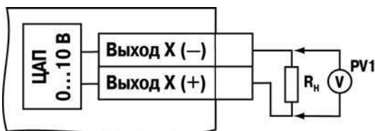
Рисунок Б.14 – Схема подключения нагрузки к ВУ типа У. R_{н} > 2 \text{ кОм}
